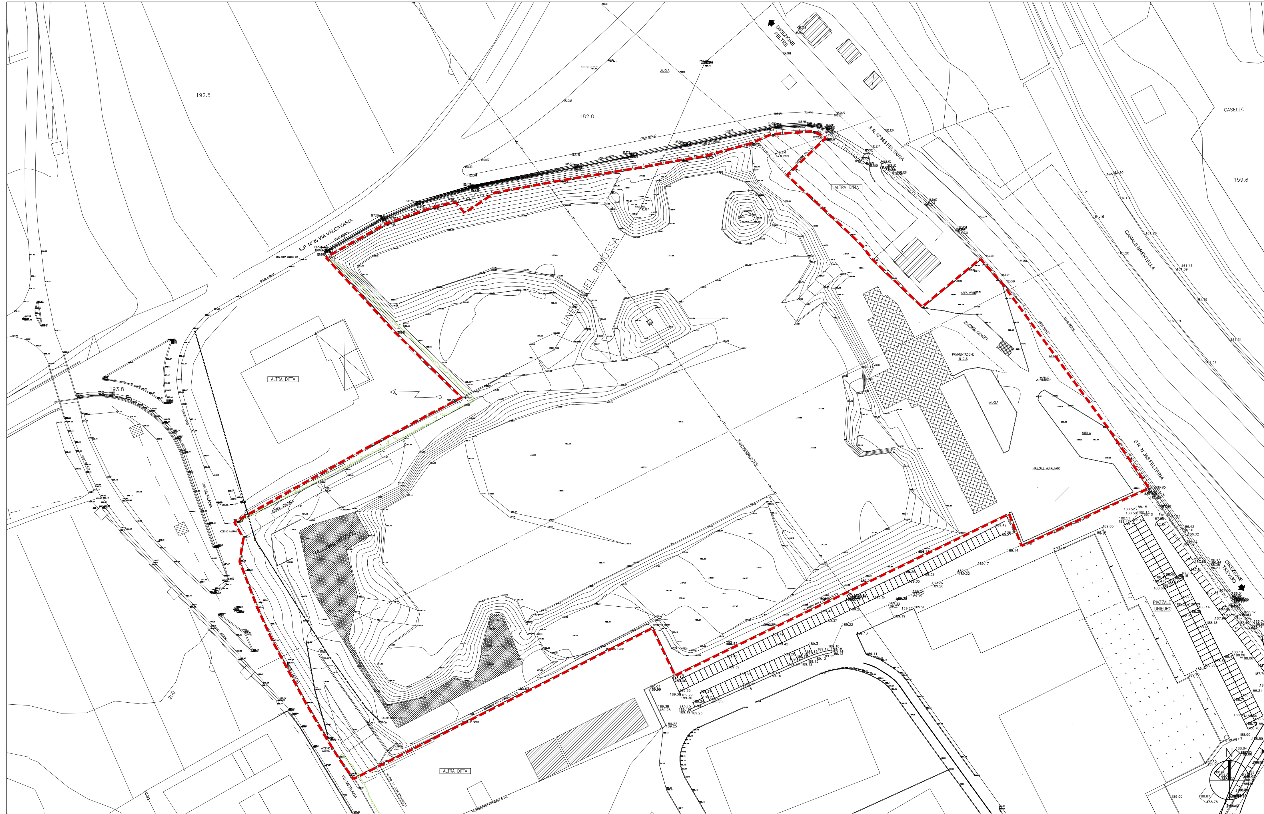
RILIEVO TOPOGRAFICO - Scala 1:1000
